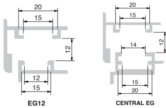
Frame groove 12
