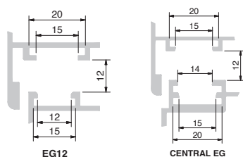
Frame groove 12
