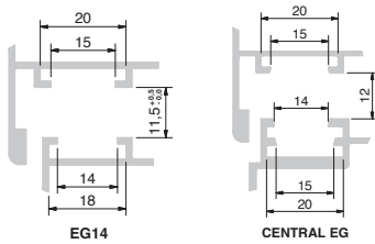
Frame groove 14
