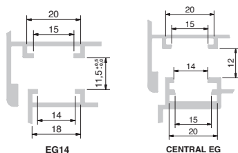
Frame groove 14
