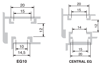
Frame groove 10
