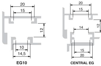
Frame groove 10
